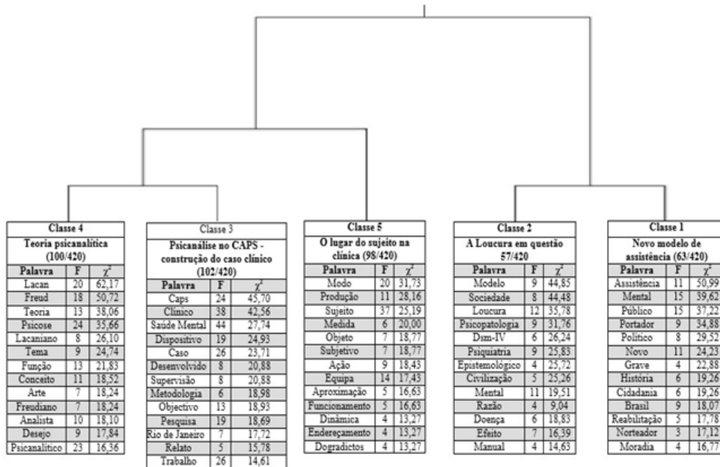
Figura 1. Dendrograma.
