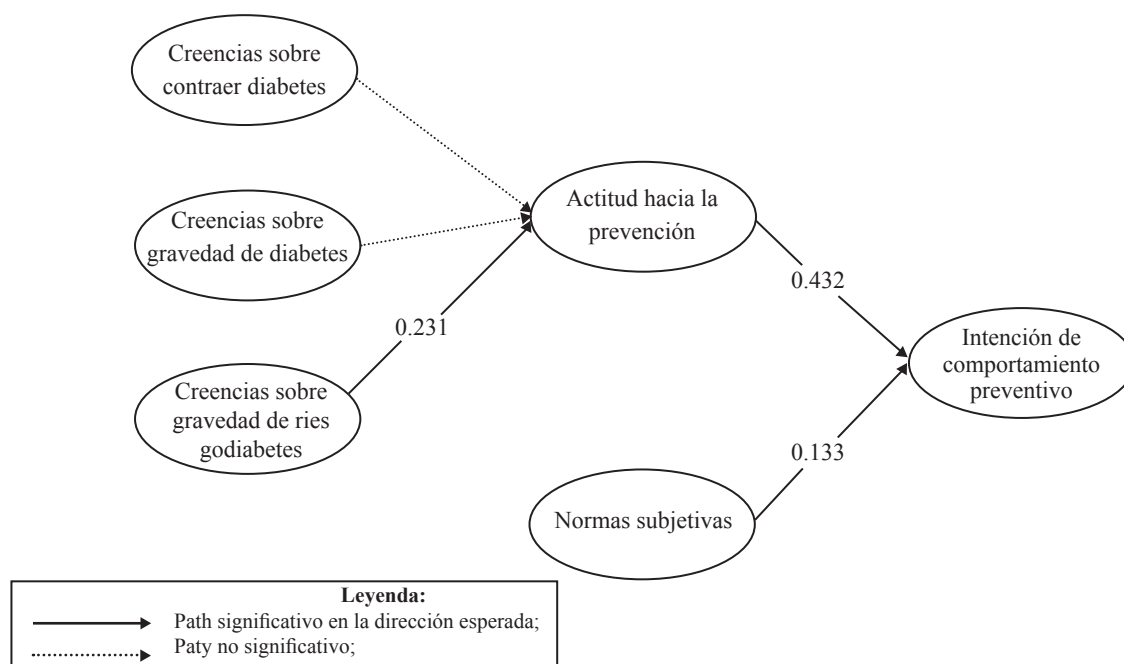
Figura 2 - Versión final del modelo de ecuaciones estructurales para predecir la ICP de diabetes en hijos de pacientes diabéticos.
